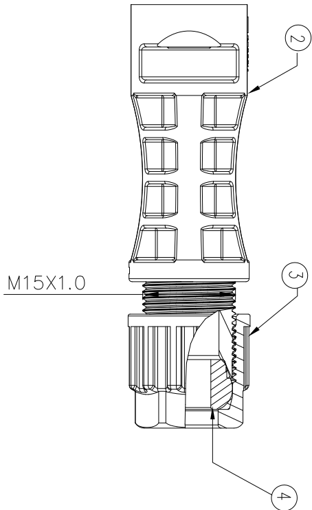
截面 B-B
